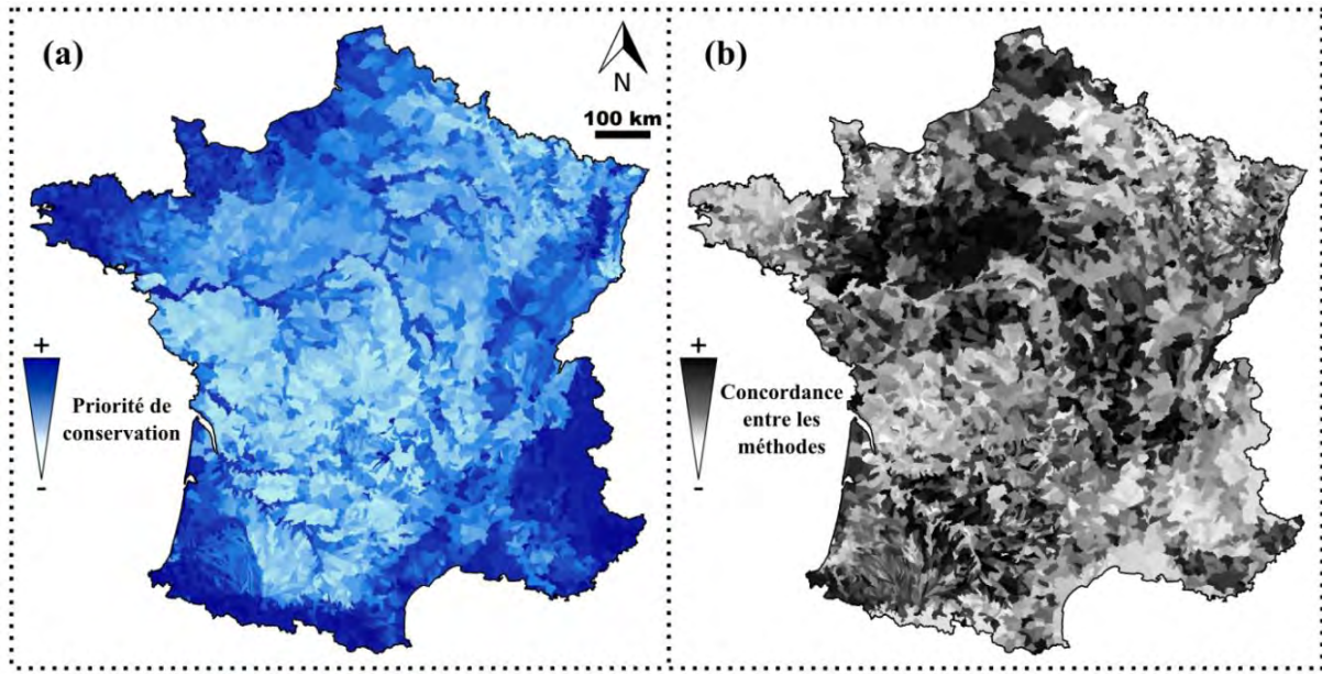
Figure 4.3. Consensus entre les priorités de conservation obtenues avec les trois méthodes de priorisation multi-objectifs considérées et concordance entre les trois méthodes. (a) Les valeurs du consensus (i.e. la moyenne des priorités de conservation obtenues avec les trois méthodes ; cf. Figure 4.1 ) sont représentées au moyen d'un gradient allant du bleu clair (priorités faibles) au bleu foncé (priorités élevées). (b) La concordance entre les priorités de conservation obtenues avec les trois méthodes est représentée au moyen d'un gradient de gris allant du blanc (fortes valeurs de RMSE indiquant une faible concordance entre les méthodes) au noir (faibles valeurs de RMSE indiquant que les trois méthodes fournissent des priorités de conservation très proches).
